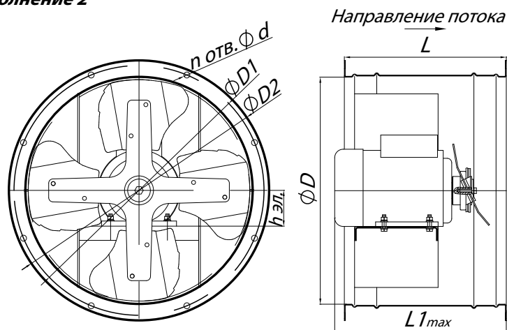
Исполнение 2
