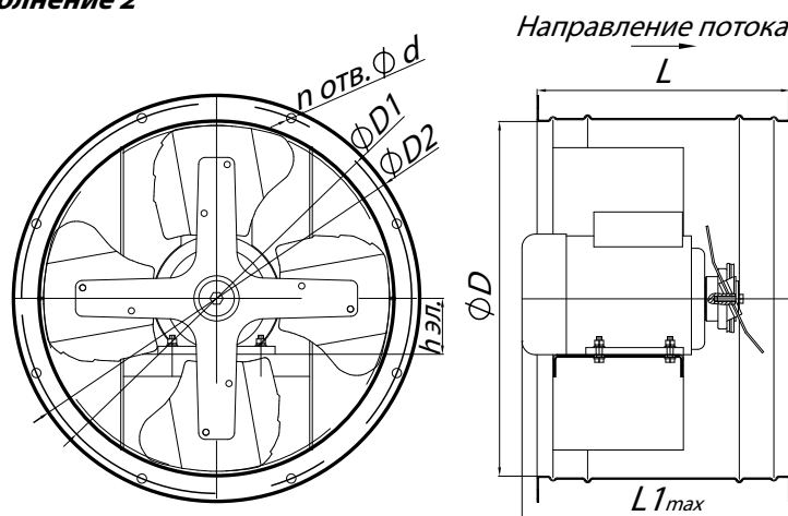
Исполнение 2
