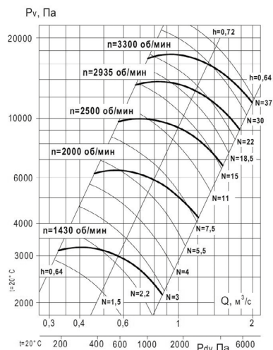
Аэродинамическая характеристика вентилятора ВР 140-15-8 исп. 1 и 5
