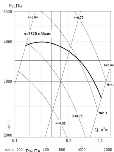
Аэродинамическая характеристика вентилятора ВР 140-15-4,5 исп. 1
