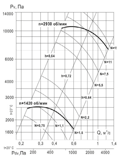
Аэродинамическая характеристика вентилятора ВР 140-15-7,1 исп. 1
