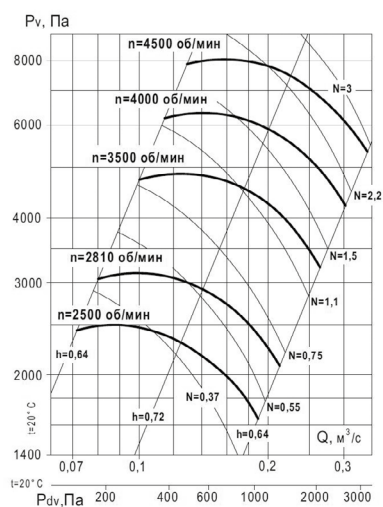
Аэродинамическая характеристика вентилятора ВР 140-15-4 исп. 1 и 5
