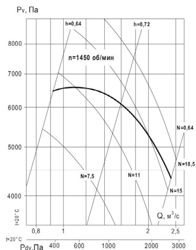
Аэродинамическая характеристика вентилятора ВР 140-15-11,2 исп. 1
