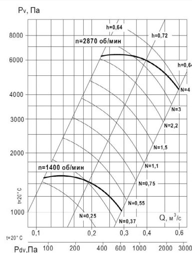
Аэродинамическая характеристика вентилятора ВР 140-15-5,6 исп. 1
