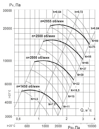
Аэродинамическая характеристика вентилятора ВР 140-15-10 исп. 1 и 5
