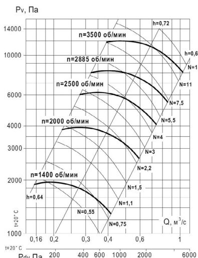
Аэродинамическая характеристика вентилятора ВР 140-15-6,3 исп. 1 и 5
