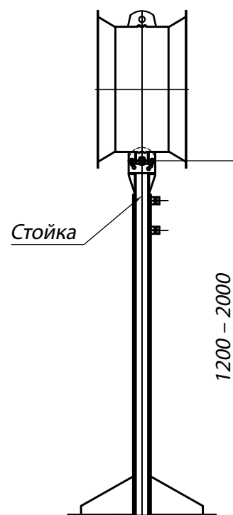
Крепление на стойке
