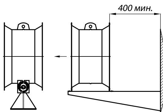
Крепление на кронштейнах.
